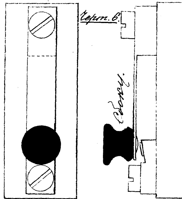
Поворотный коммутаторъ.
